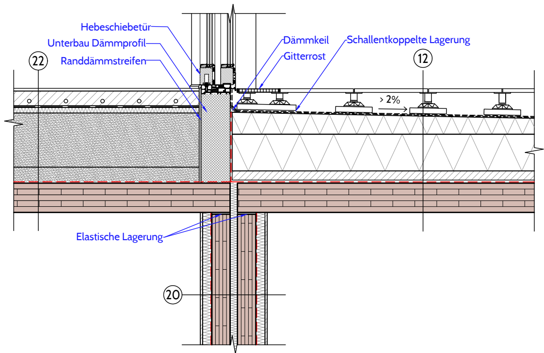
Schnitt B-B M 1:20
