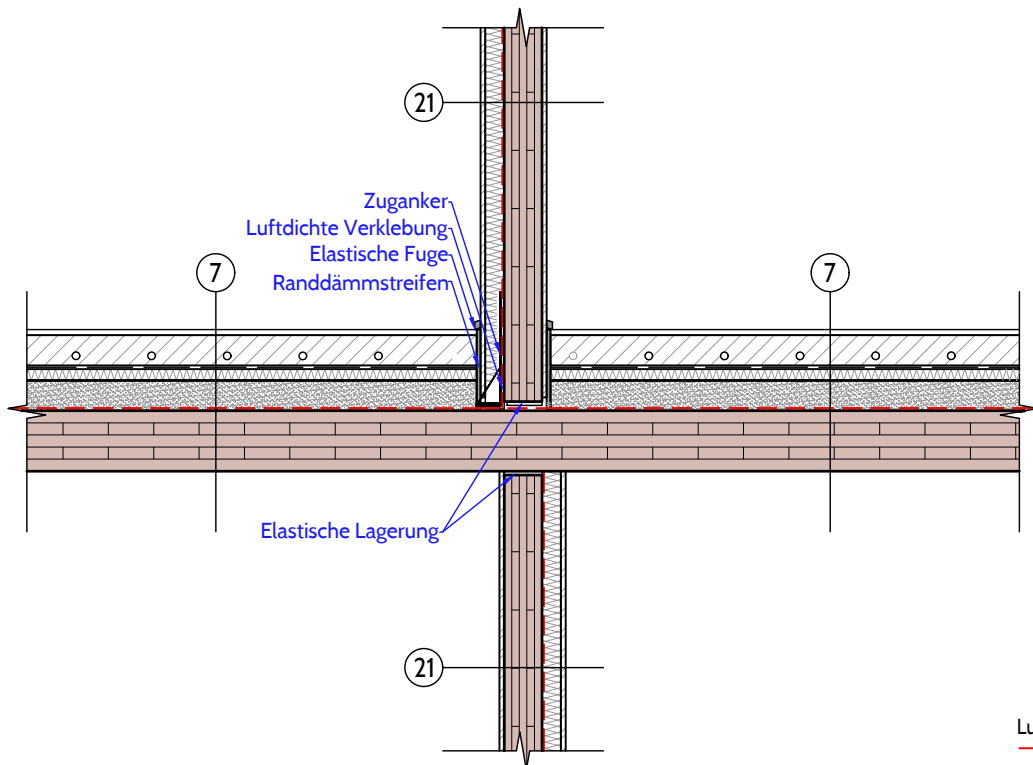
Schnitt B-B M 1:20
